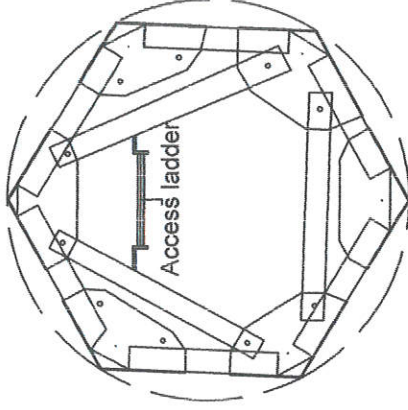
SECTION B-B' E 1:15
